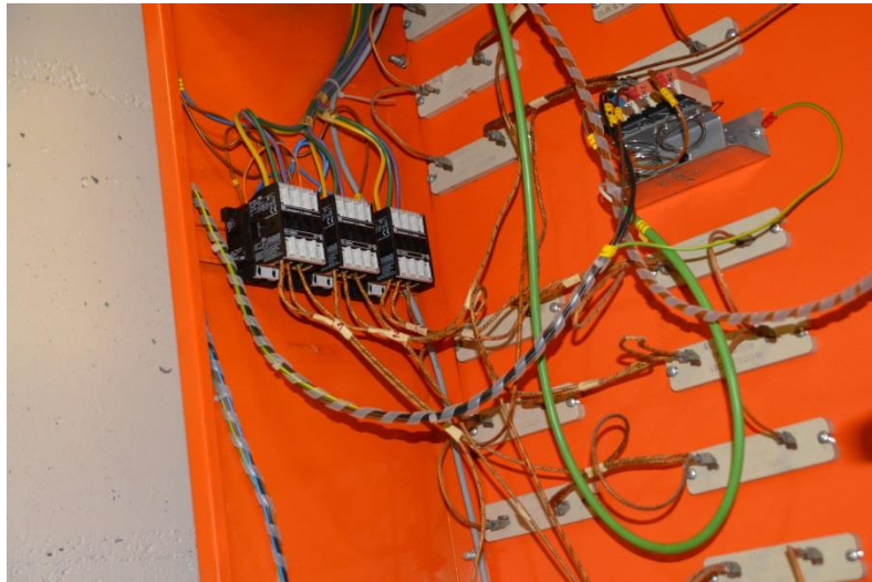
Neue Lastschützen mit neuer Verdrahtung
